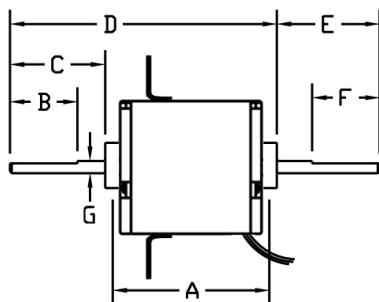
NEMA 42
