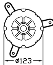
NEMA 42
